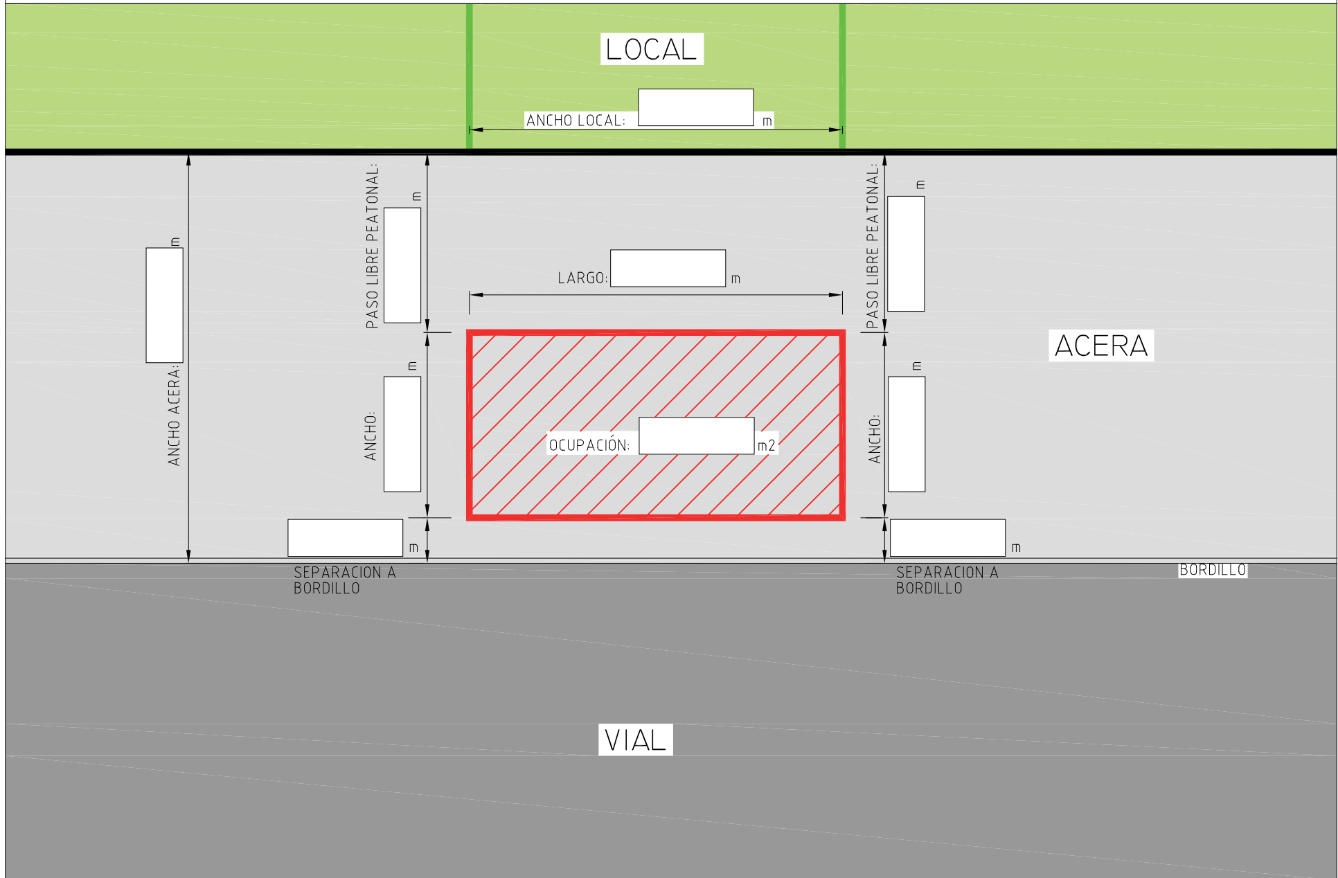
CROQUIS 2: OCUPACION COLINDANTE CON CALZADA
